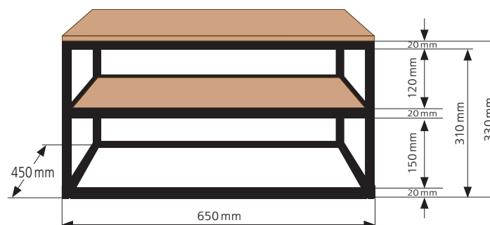
Konferenční stůl – Výkres pro cenovou nabídku
