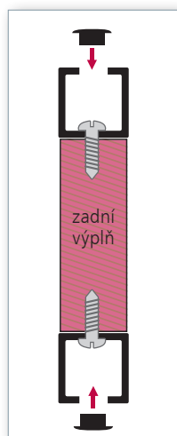
VARIANTY HORNÍHO UCHYCENÍ
