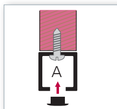
VARIANTY SPODNÍHO UCHYCENÍ
