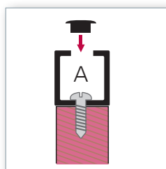
VARIANTY HORNÍHO UCHYCENÍ
